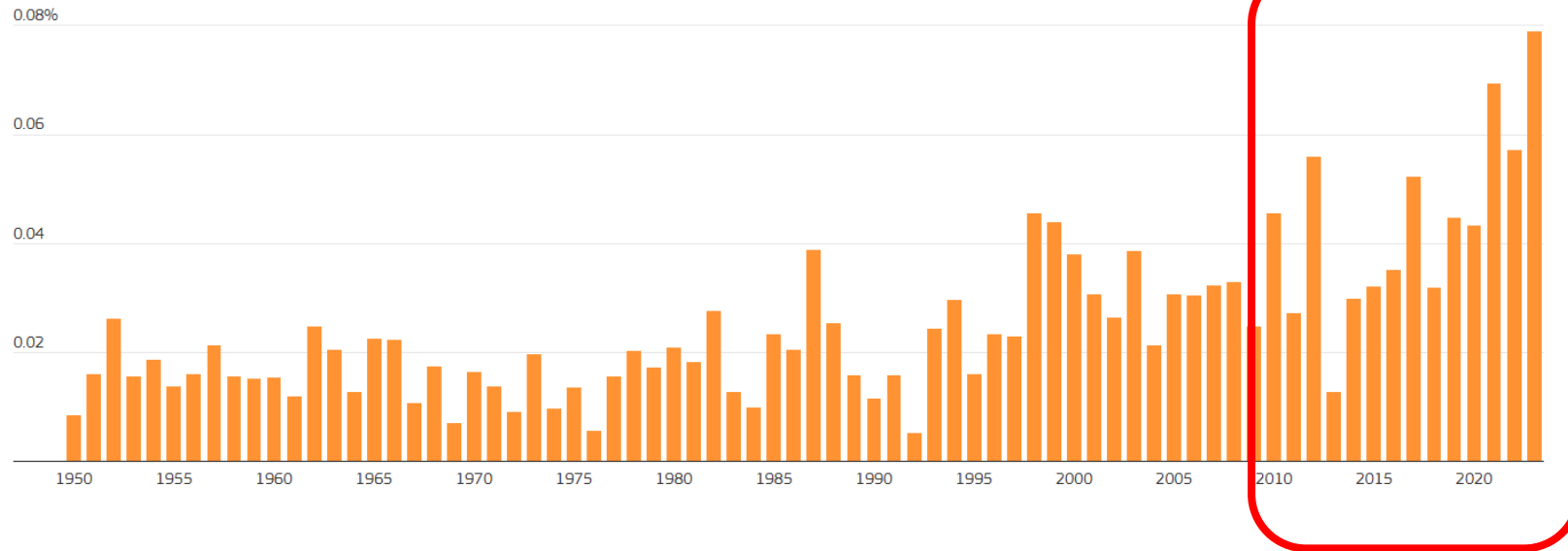
Percentuale di giorni con stress termico estremo in Europa (dal 1950 al 2023)
