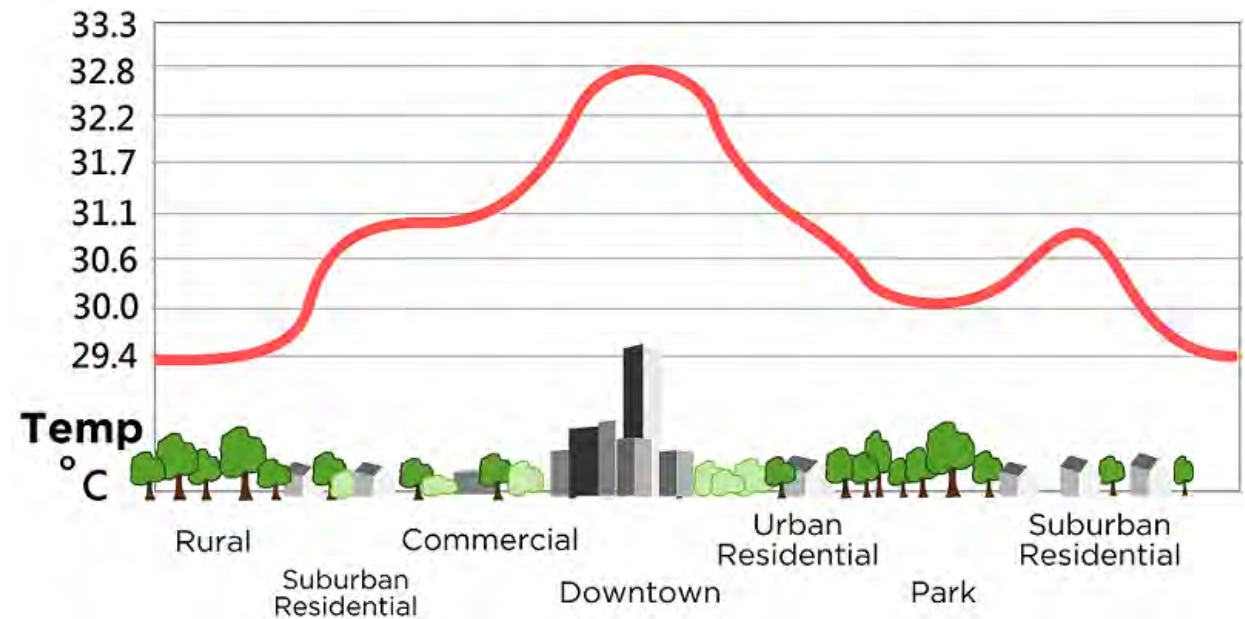
Profilo tipico delle temperature isola di calore
