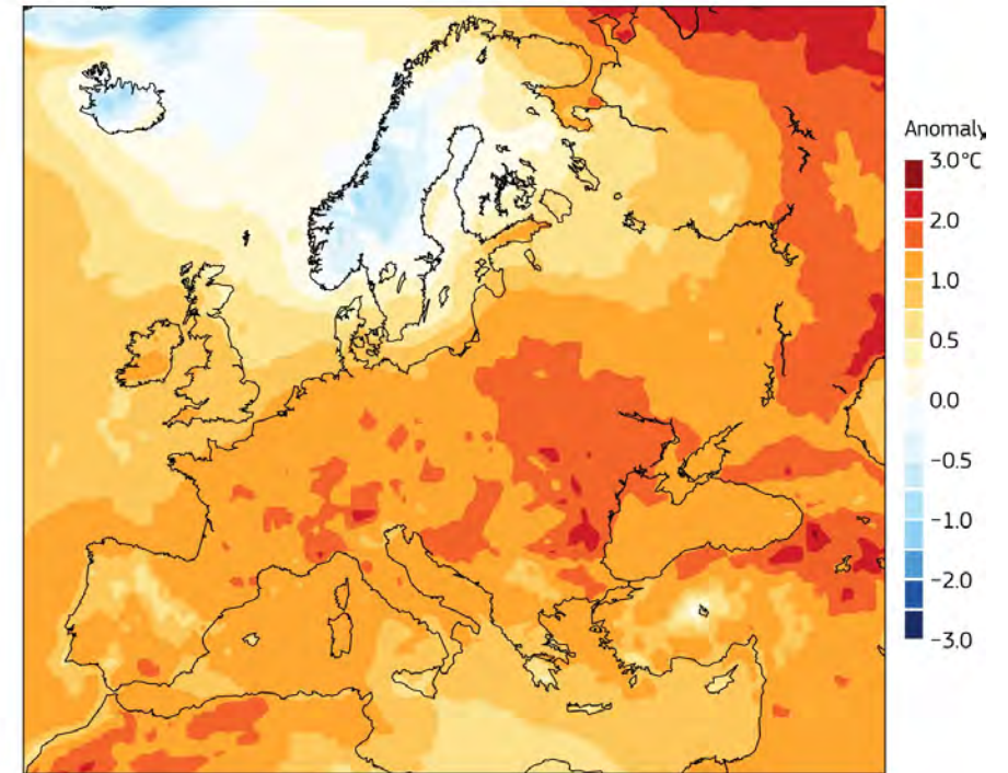
Temperatura superficiale media (2023 vs 1991-2020)
